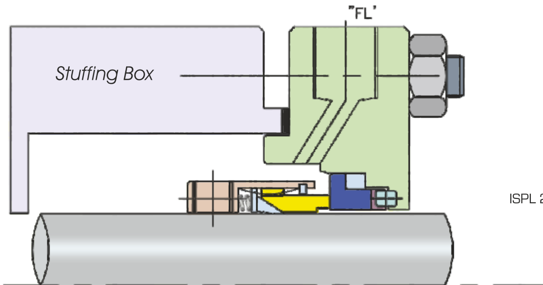
ISPL-2403 Multi Spring UB Wedge Type
