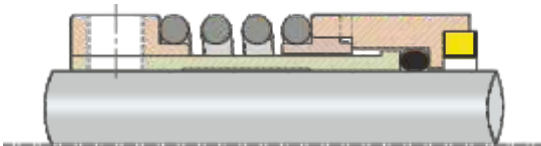
ISPL-2406A Slip Type Seal
