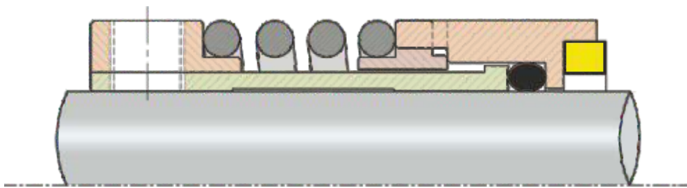
ISPL-2406A Slip Type Seal
