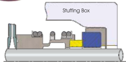
ISPL-2412 F Long Bellow Type MG12
