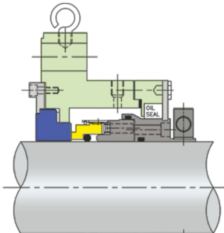
ISPL 24555 B GLR Seal
